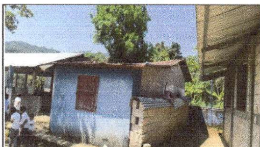
FOTO 9: Sustitución de lámina, por lámina troquelada aluzinc calibre 26 Y Sustitución de estructura de soporte de madera, por metal
